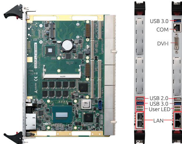
cPCI-6530(BL) cPCI-6530(BL)V
